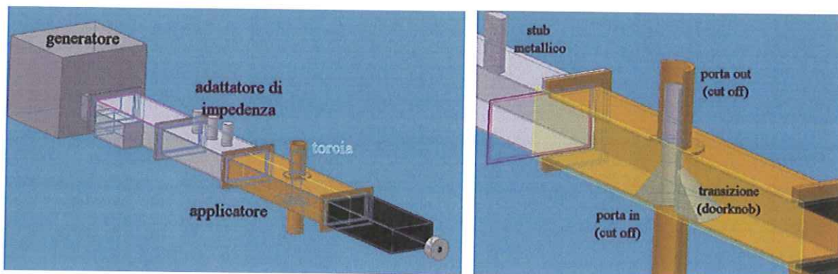
Successive iterazioni della simulazione numerica hanno portato alla definizione di massima della geometria dell'applicatore a microonde.
